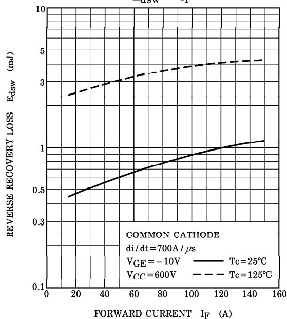
E_{dsw} - I_F
